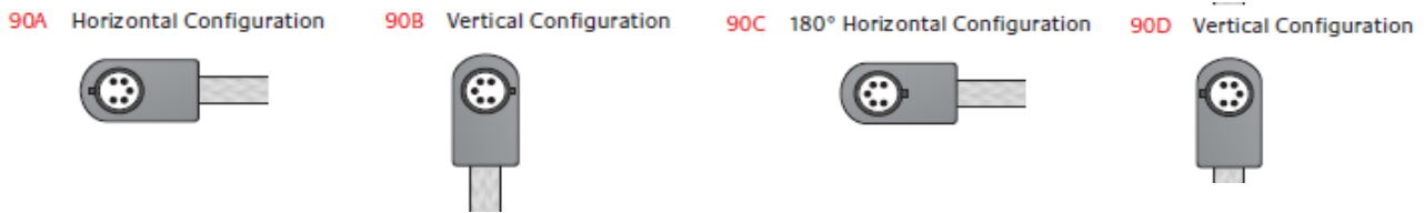
orientamento dei PIN nei connettori a 90° per i cavi per braccio (vista frontale)
